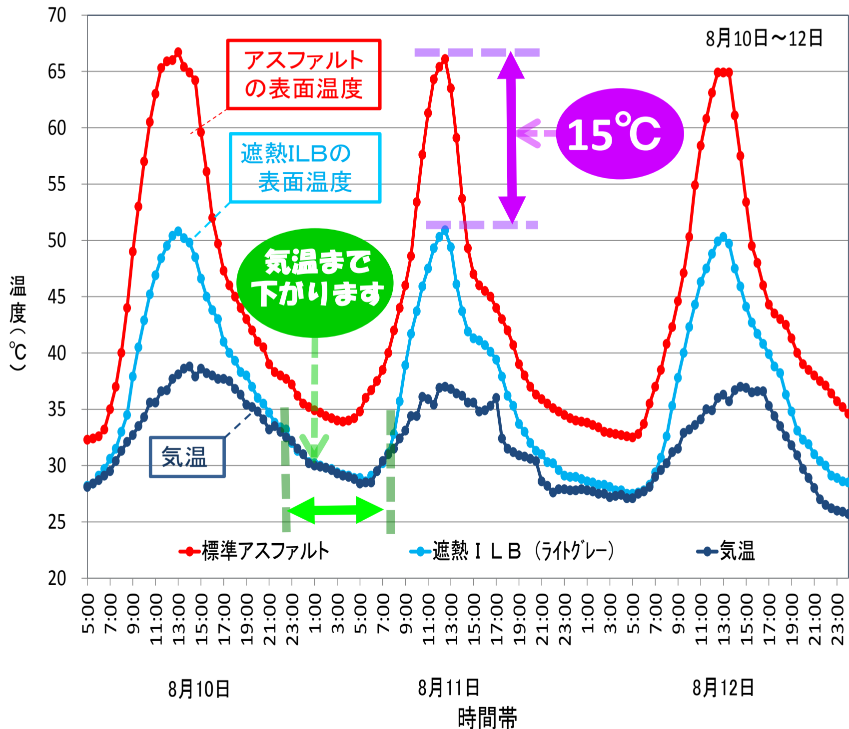
図. 温度測定結果(8月10日~12日)
